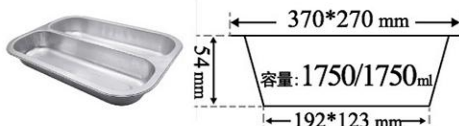
BP370/6200-F 100只/箱
